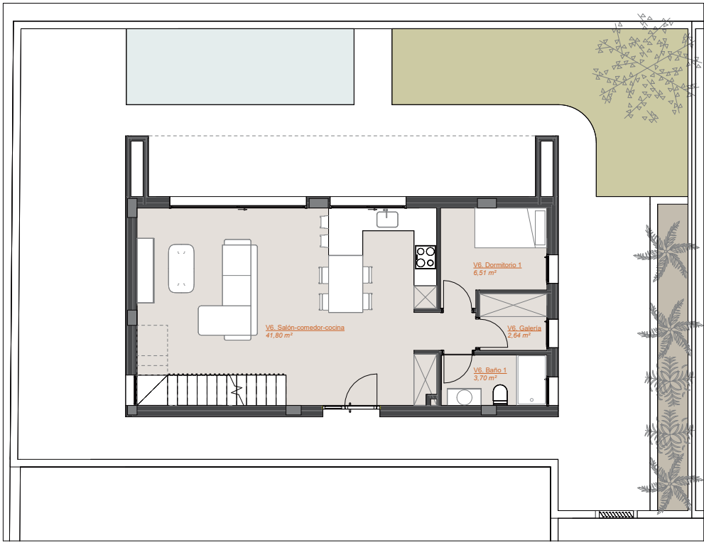
Planta baja. Vivienda 06
