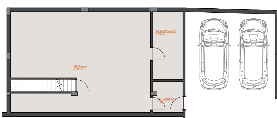
Planta sótano. Vivienda 06 E / 1 : 100
