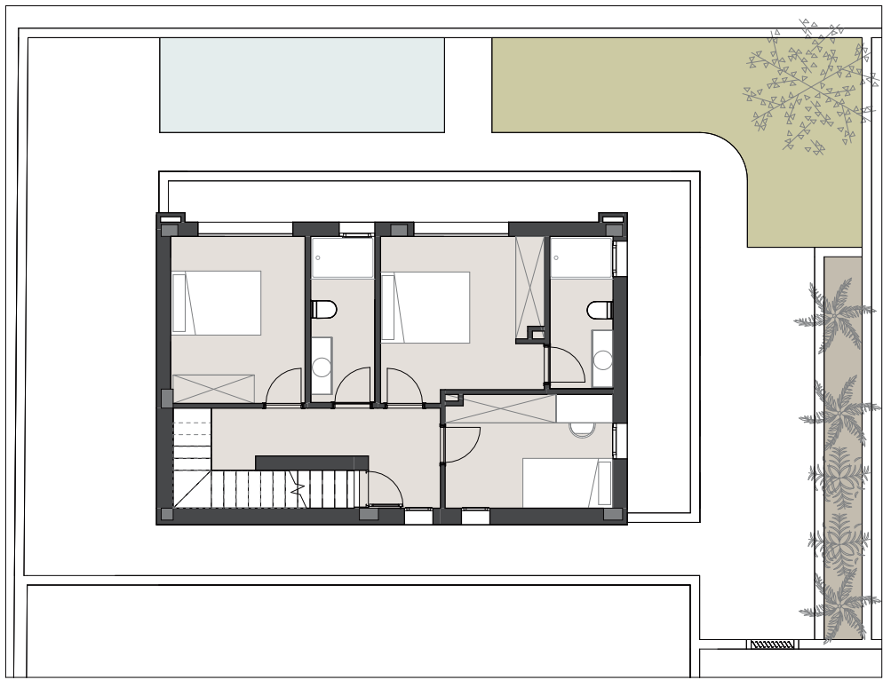
Planta Primera. Vivienda 06
