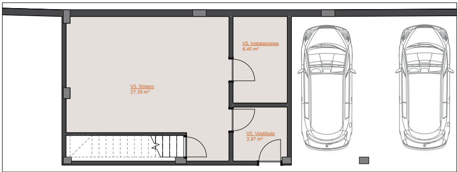
Planta sótano. Vivienda 05
