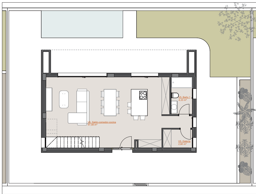
Planta baja. Vivienda 05 E / 1 : 100
