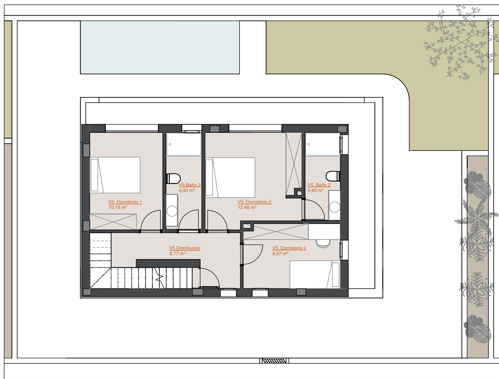
Planta Primera. Vivienda 05 E / 1 : 100
