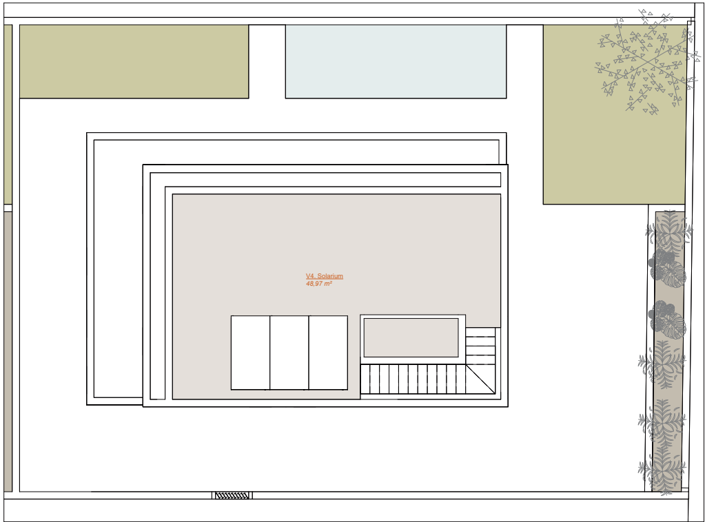
Planta cubierta. Vivienda 04 E / 1 : 100
