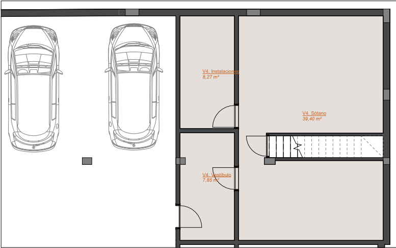
Planta sótano. Vivienda 04
