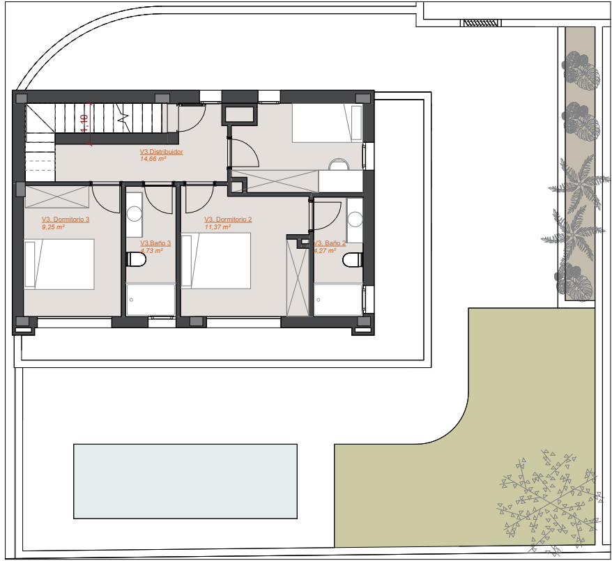
Planta Primera. Vivienda 03 E / 1 : 100
