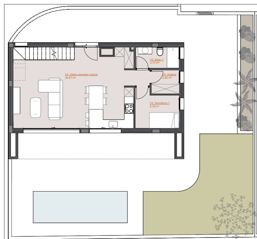
Planta baja. Vivienda 03 E / 1 : 100
