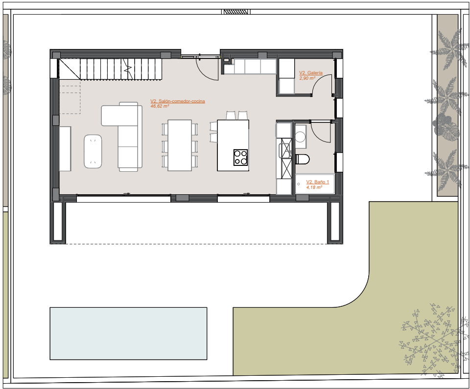
Planta baja. Vivienda 02
